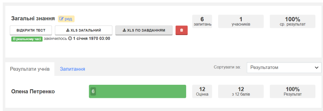
Рис. 17. Результати тестування
