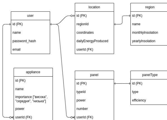
Рисунок 3.1 – UML-діаграма бази даних
