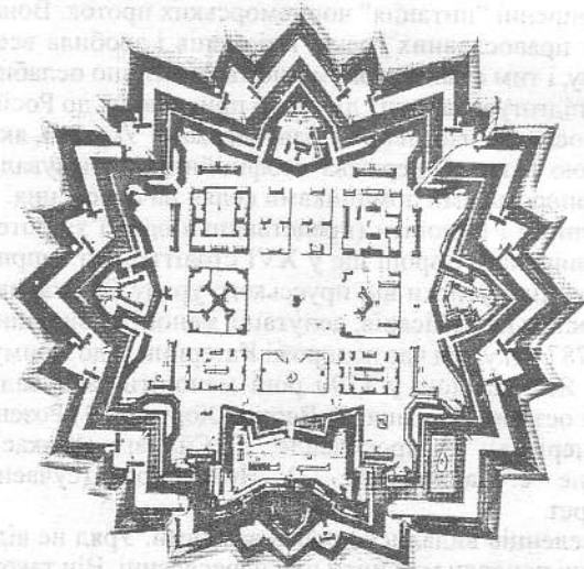
План Олександрівської фортеці (1771 рік)
