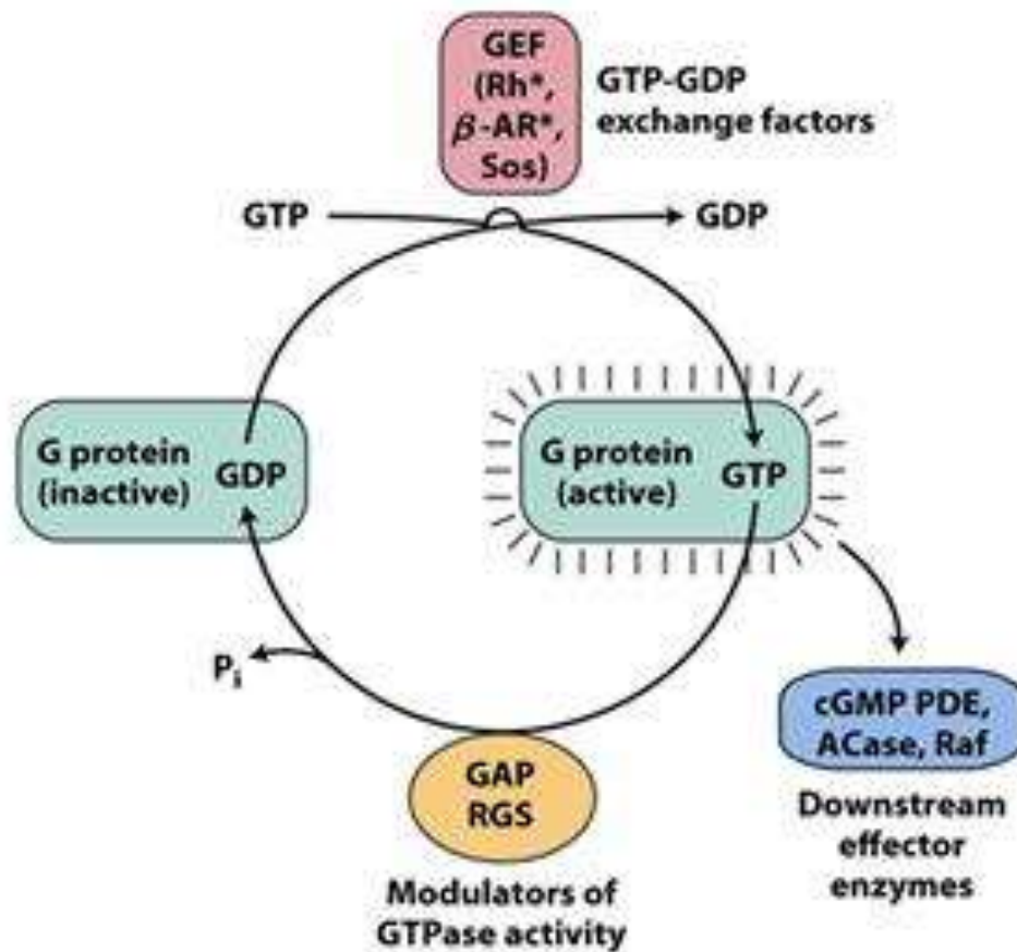
Рис. 35 Регулювання активації та інактивації G-білка
