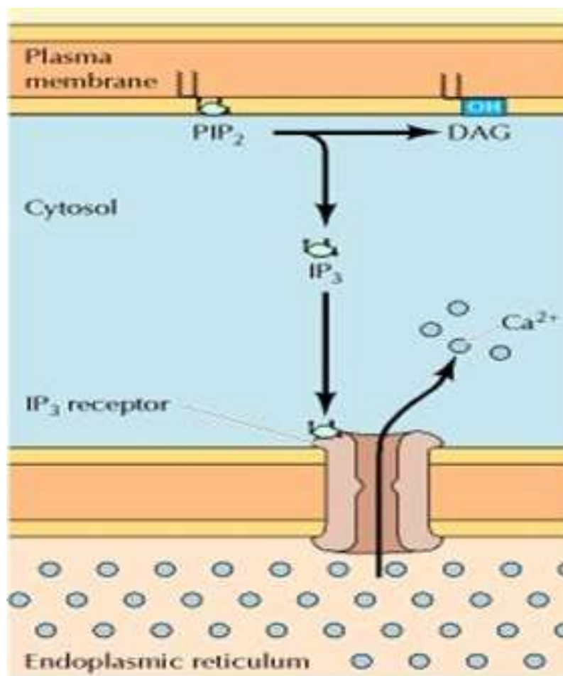
Рис. 29 Мобілізація \text{Ca}^{2+} за допомогою IP 3
