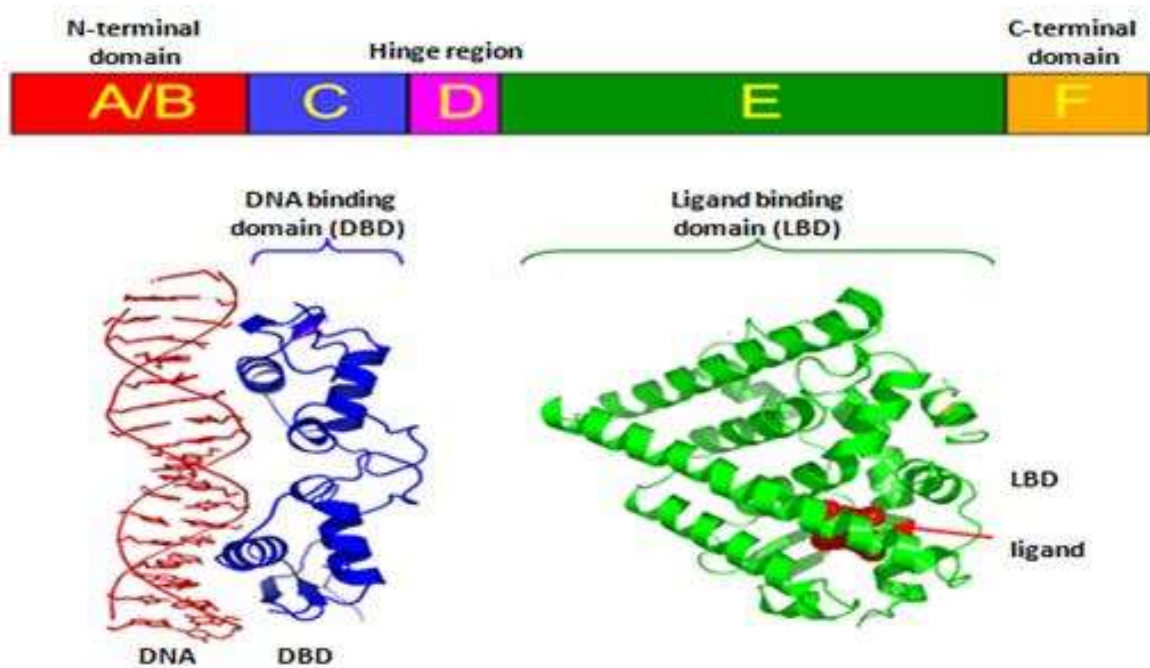
Рис. 11 Структурна організація ядерних рецепторів (рецептор естрогену)
