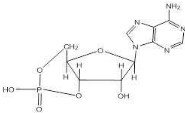
Рис. 16 Циклічний аденозинмонофосфат або 3'-5'-циклічний аденозинмонофосфат
