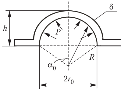
Рис. П.41. Сферическая крышка под внутренним давлением
