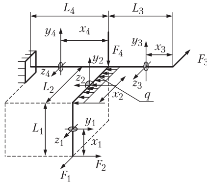
Рис. П.23. Схема нагружения пространственного стержня
