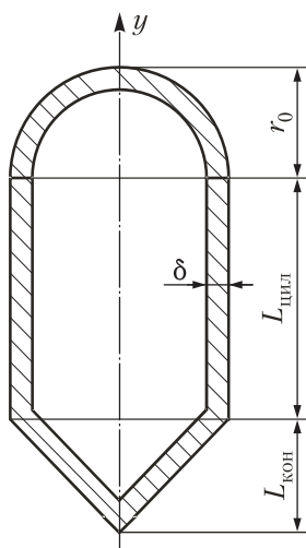
Рис. П.39. Схема цилиндрической оболочки
