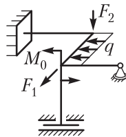
Рис. П.27. Схема пространственной рамы
