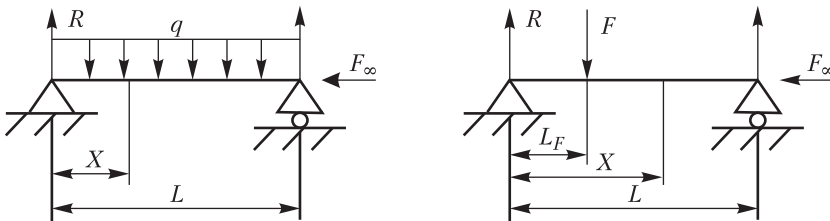
Рис. П.32. Расчетные схемы нагружения балок
