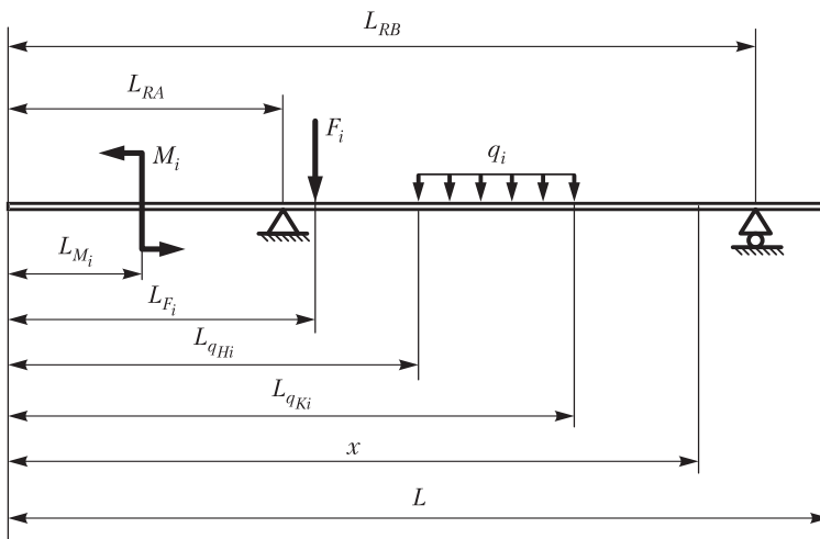
Рис. П. 11. Условная схема нагружения балки на двух опорах
