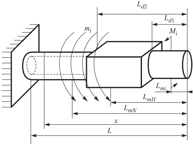
Рис. П. 16. Условная схема нагружения ступенчатого стержня
