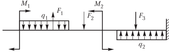
Рис. П.18. Схема нагружения консольной балки
