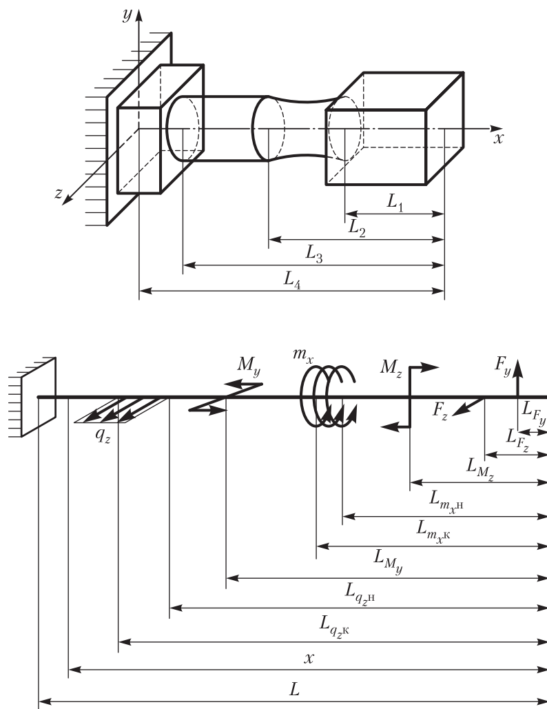
Рис. П.22. Стержень переменного сечения (вверху) и условная схема его нагружения (внизу)
