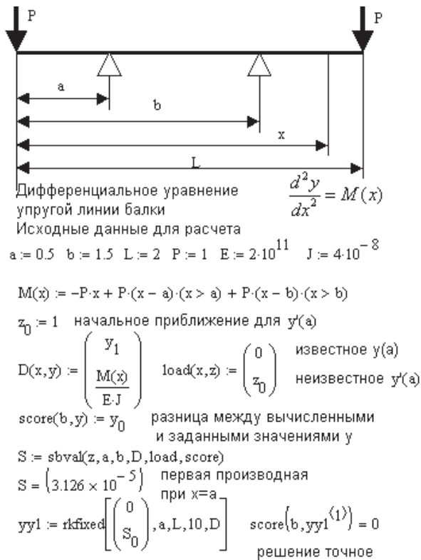
Рис. 6.25. Расчет прогиба балки функциями sbval и rkfixed
