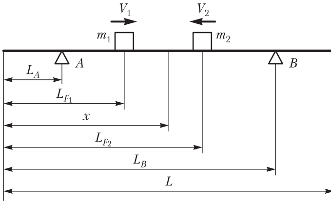
Рис. П.5. Схема движения двух машин по мосту
