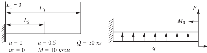
Рис. П.43. Балка, граничные условия и нагрузки на балку
