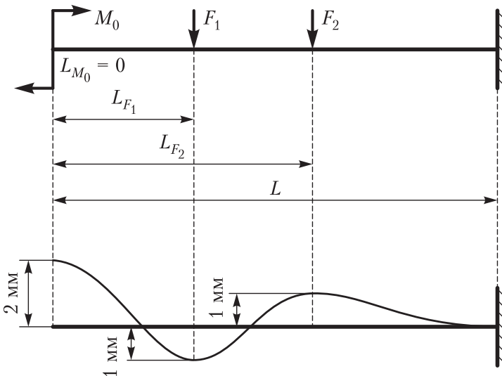
Рис. П.42. Перемещения консольной балки и нагрузки, которые надо определить
