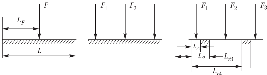
Рис. П.20. Схемы балок на упругом основании
