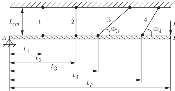
Рис. П.14. Растяжение шарнирно-стержневой системы
