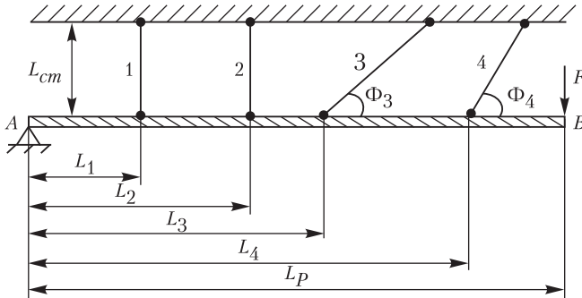
Рис. П.21. Схема шарнирно-стержневой системы
