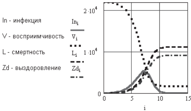
Рис. 3.23. Рекурсивные вычисления в модели распространения инфекции
