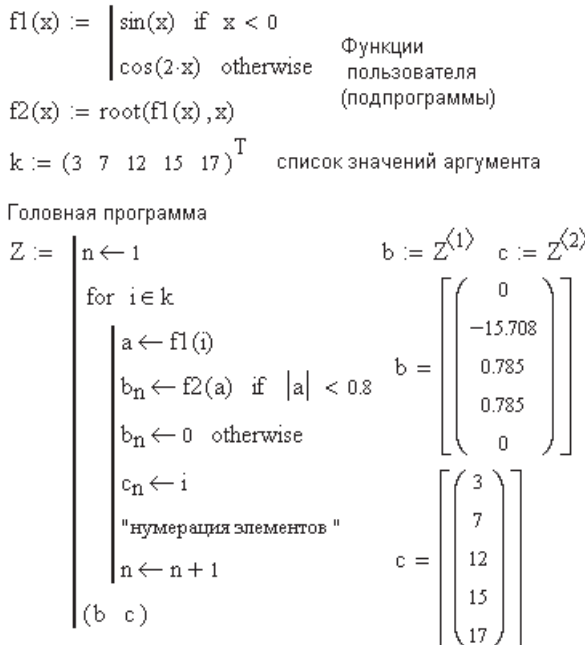
Рис. 9.12. Вложенные подпрограммы
