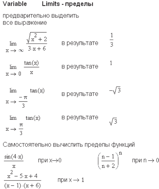
Рис. 5.10. Примеры вычисления пределов функций
