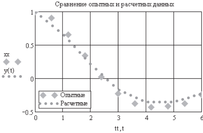
Рис. 9.25. Результаты решения ОДУ (см. рис. 9.23)
