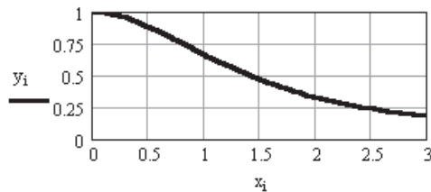
Рис. 6.12. Решение дифференциального уравнения с переменным шагом
