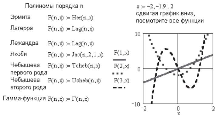
Рис. 12.31. Примеры использования ортогональных полиномов
