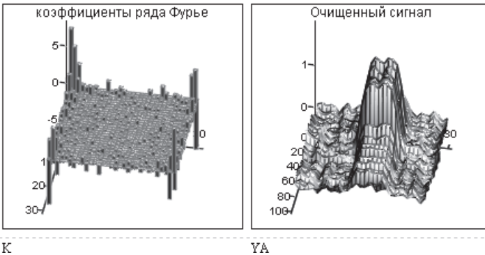
Рис. 7.25. Двухмерное преобразование Фурье массива данных с помехами (см. рис. 7.24)
