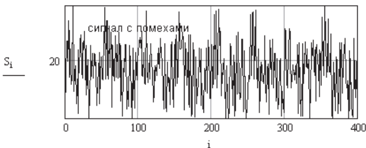
Рис. 18.4. График сигнала, требующего очистки от помех
