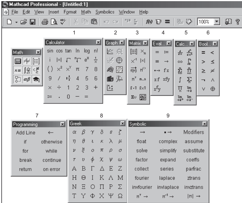
Рис. 1.4. Математическая панель
