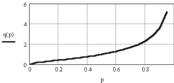
Рис. 8.6. График определения квантиля вероятности q
