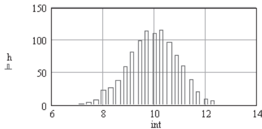
Рис. 8.9. Применение функции histogram
