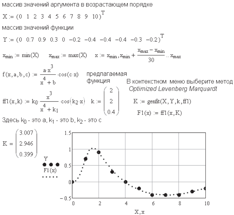
Рис. 7.19. Применение функции genfit без вычисления производных в Mathcad 13
