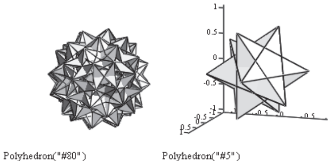
Рис. 15.22. Примеры построения поверхностей многогранников
