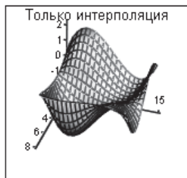
Рис. 12.14. Результаты преобразования матрицы M (см. рис. 12.13) в функцию
