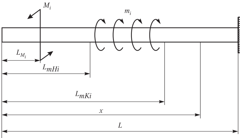
Рис. П.9. Условная схема кручения стержня
