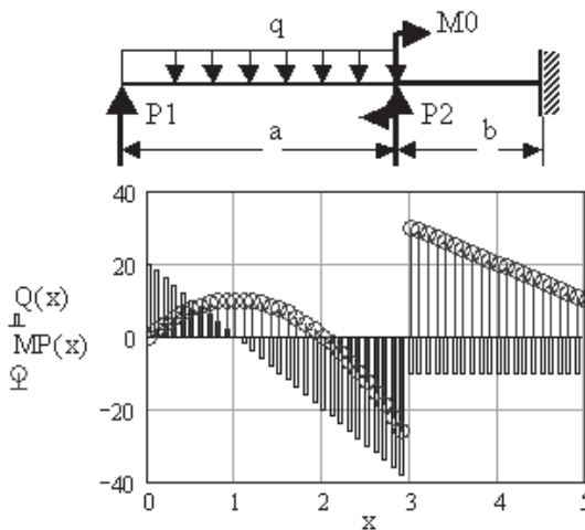
Рис. 9.4. Эпюры поперечной силы и изгибающего момента при изгибе балки (см. рис. 9.3)
