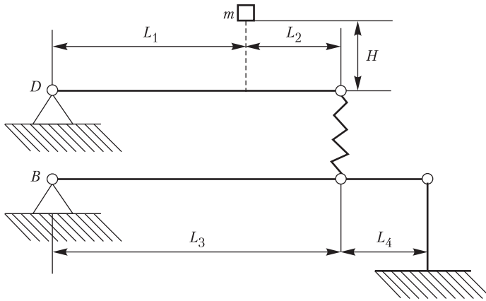
Рис. П.35. Схема ударного нагружения сложной системы
