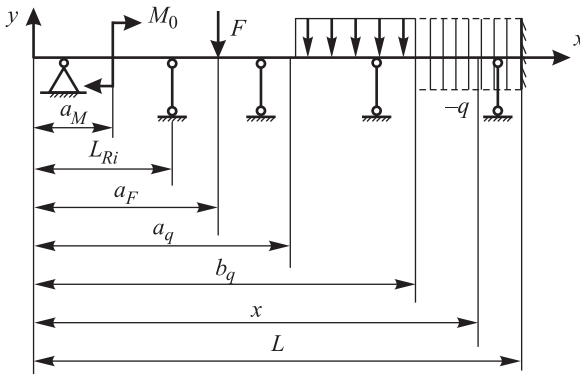
Рис. П.29. Схема многопролетной балки
