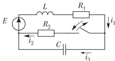
Рис. П.4. Схема электрической цепи
