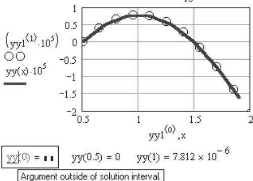
Рис. 6.26. Определение прогиба балки (см. рис. 6.25) функцией Odesolve
