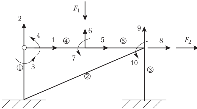
Рис. П.45. Разбивка плоской рамы на конечные элементы и нумерация перемещений в ней
