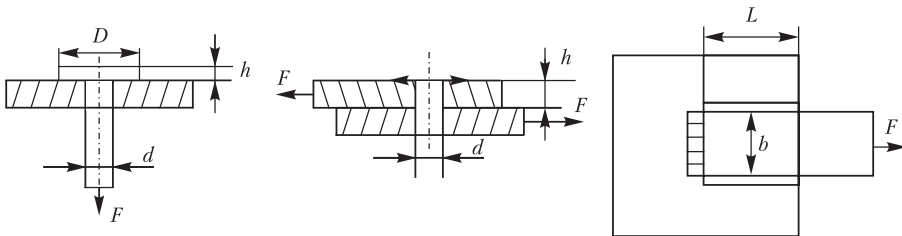
Рис. П.15. Схемы для расчета тяги, штифта и сварного соединения
