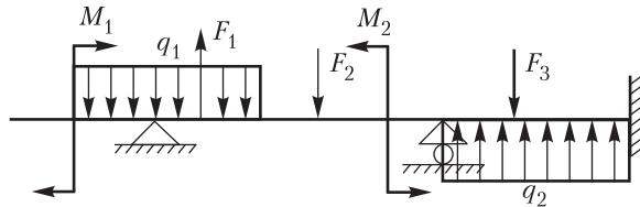
Рис. П.19. Расчетная схема балки на двух опорах
