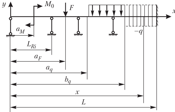
Рис. П.28. Схема многопролетной балки с заделкой
