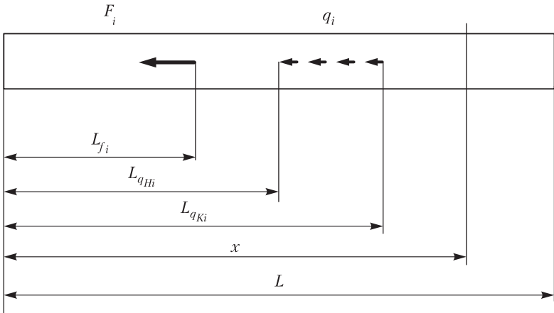
Рис. П.8. Условная схема растяжения стержня
