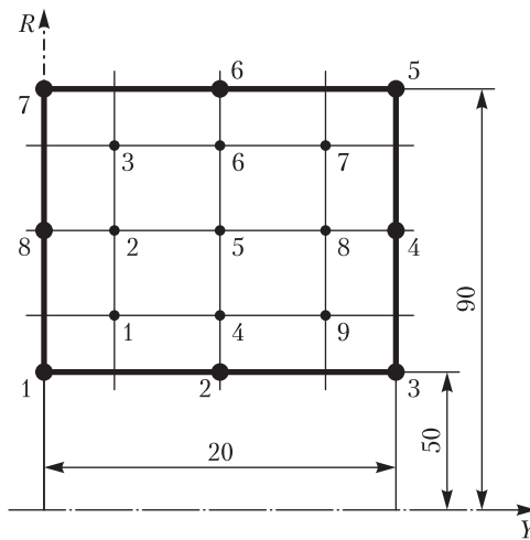
Рис. П.49. Прямоугольный квадратичный элемент с восемью узлами и девятью точками интегрирования
