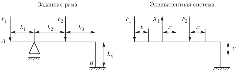
Рис. П.26. Расчетные схемы рамы
