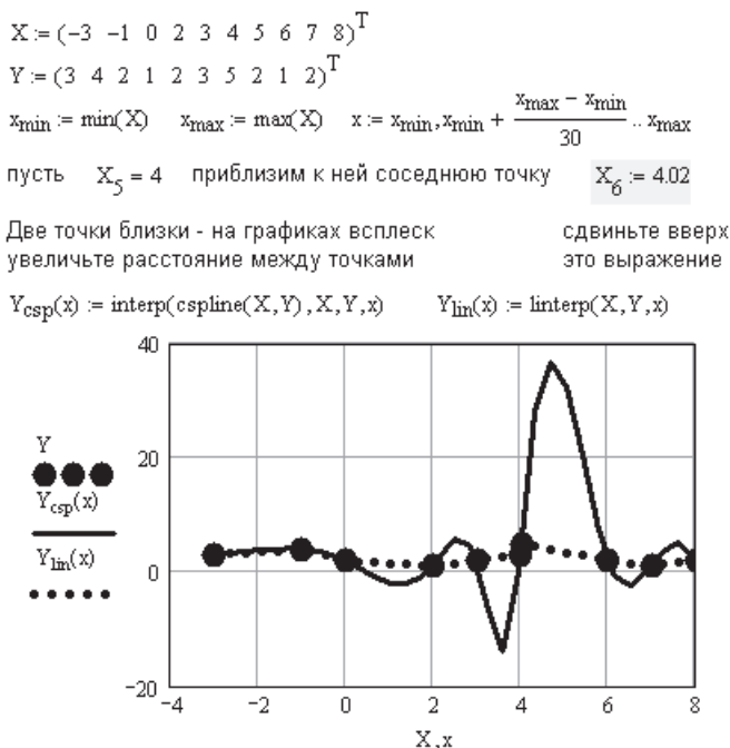
Рис. 7.4. Влияние близких точек на результат интерполяции. Массив Y приведен на рис. 7.1
