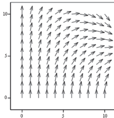
Рис. 15.25. Векторное поле функции, проекции которой — H_1 и H_2
