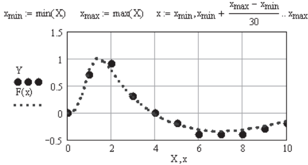
Рис. 7.17. Результаты нелинейной регрессии данных функцией genfit
