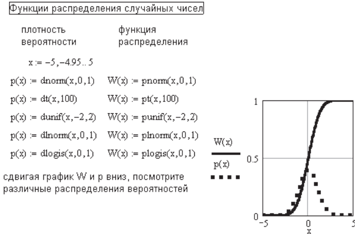
Рис. 8.5. Плотность вероятности p и функция распределения вероятностей W
