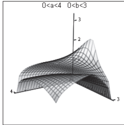
Рис. 3.12. Поверхность решений системы уравнений (см. рис. 3.11)
