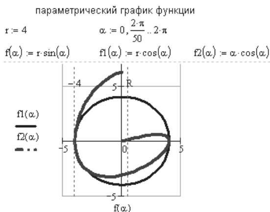
Рис. 1.14. Параметрический график функции
