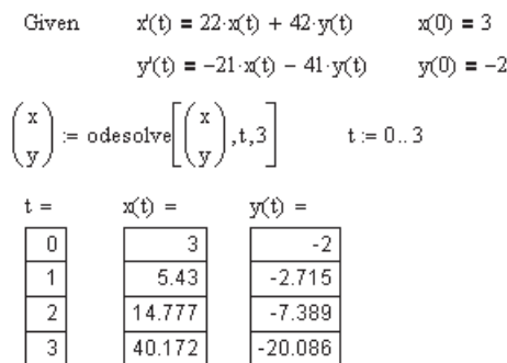
Рис. 6.21. Решение жесткой системы уравнений функцией Odesolve
