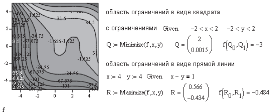
Рис. 3.21. Нахождение экстремума функции двух переменных с ограничениями
