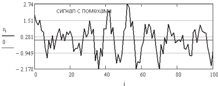
Рис. 7.22. Формирование массива зашумленных данных для последующей очистки
