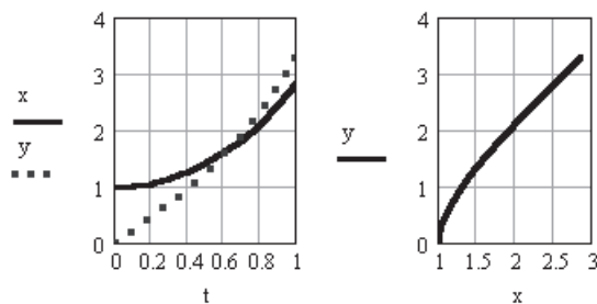
Рис. 6.15. Решение системы ОДУ первого порядка
