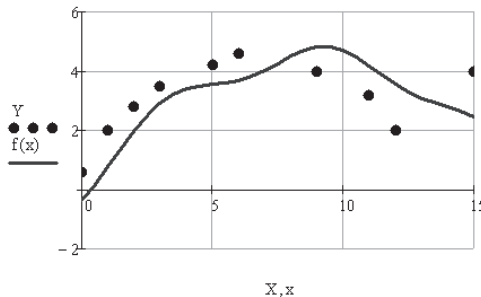
Рис. 7.14. Регрессия данных функцией linfit
