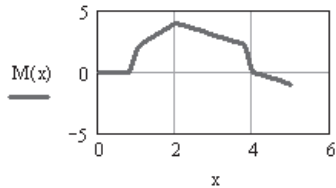
Рис. 12.24. Пример использования функции Хевисайда
