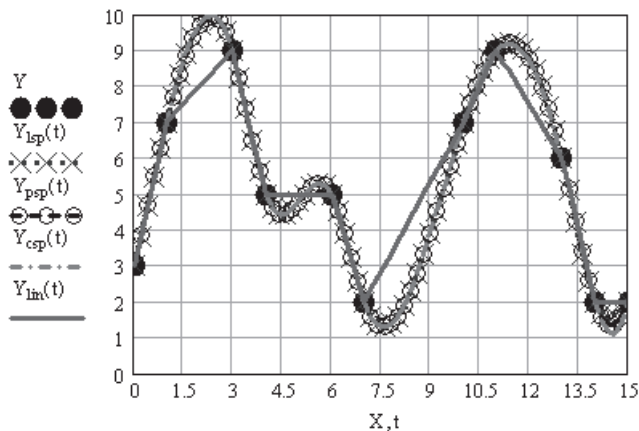
Рис. 7.2. Кубическая сплайн-интерполяция массива Y , приведенного на рис. 7.1
