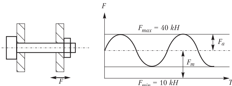
Рис. П.36. Схема болтового соединения и характеристики цикла нагружения
