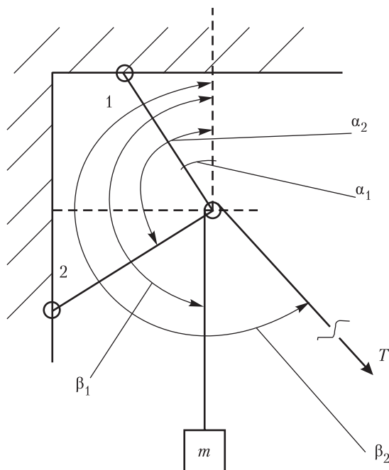
Рис. П.40. Схема нагружения кронштейна
