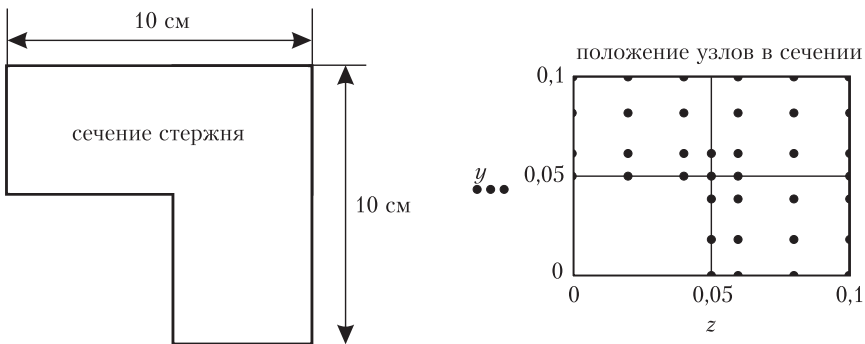
Рис. П.48. Поперечное сечение стержня и выбранные для расчета узлы
