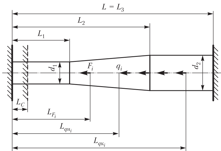
Рис. П.13. Растяжение статически-неопределимого стержня
