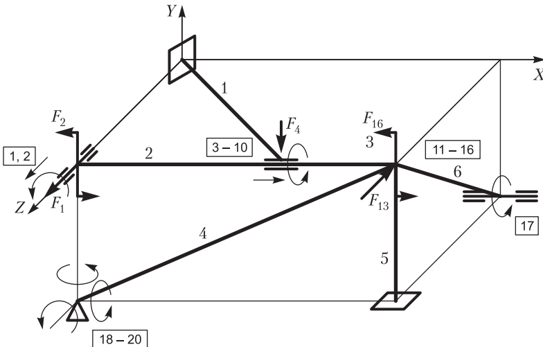
Рис. П.46. Разбивка пространственной рамы на конечные элементы и нумерация перемещений в ней
