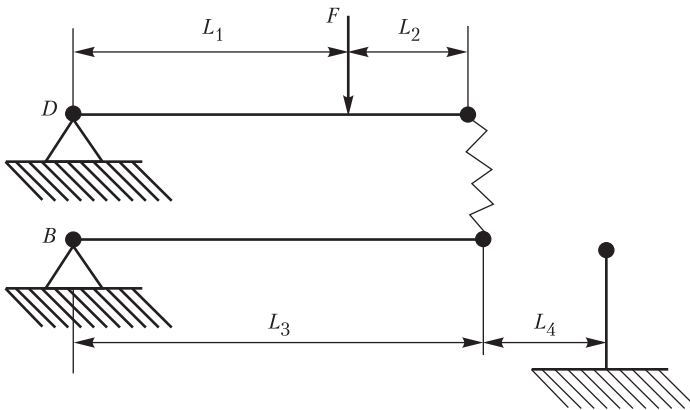
Рис. П.24. Схема нагружения сложной системы
