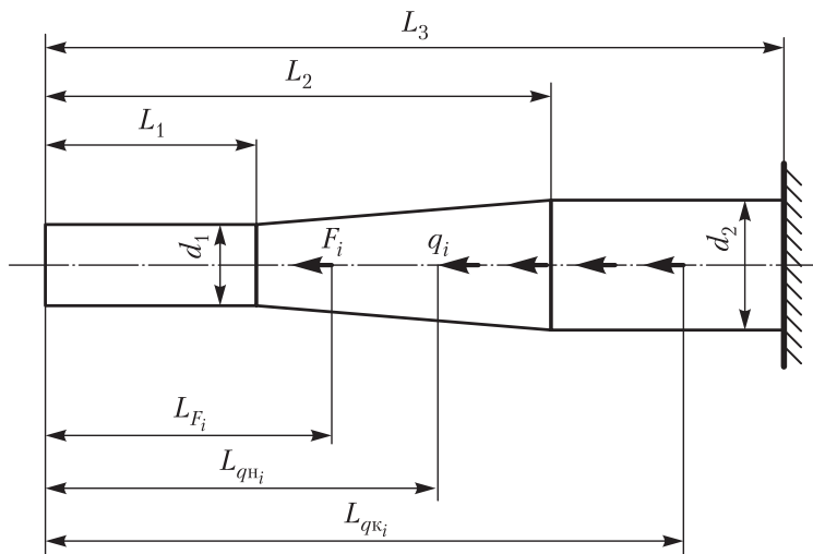
Рис. П.12. Условная схема растяжения стержня
