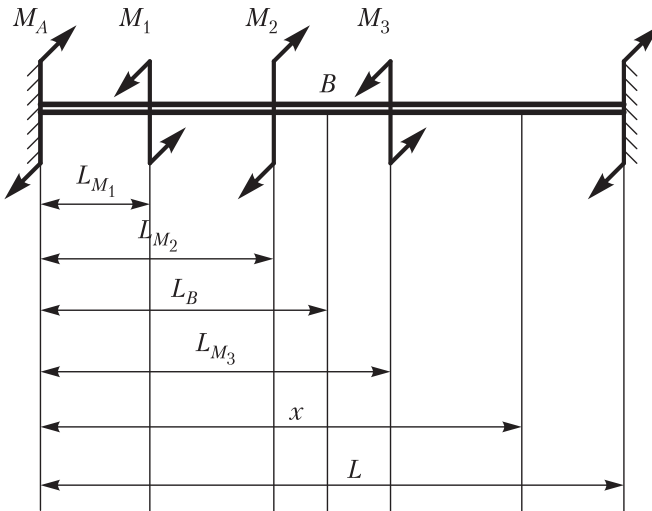
Рис. П. 17. Кручение статически-неопределимого стержня
