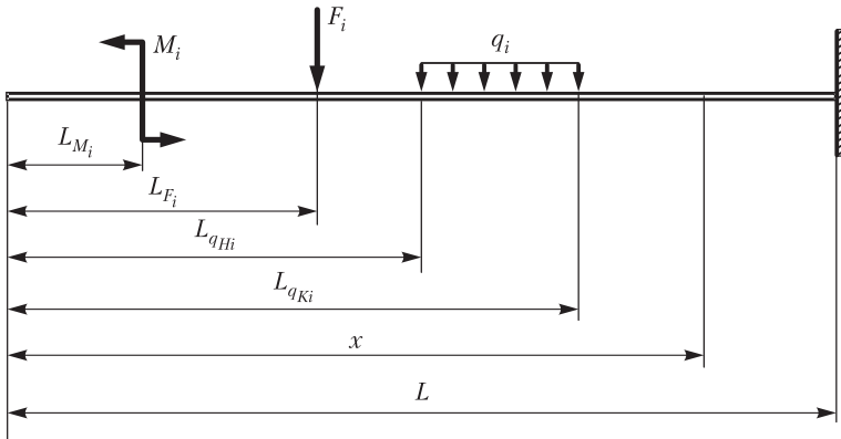
Рис. П. 10. Условная схема нагружения консольной балки
