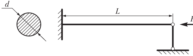
Рис. П.30. Схема сжатого стержня
